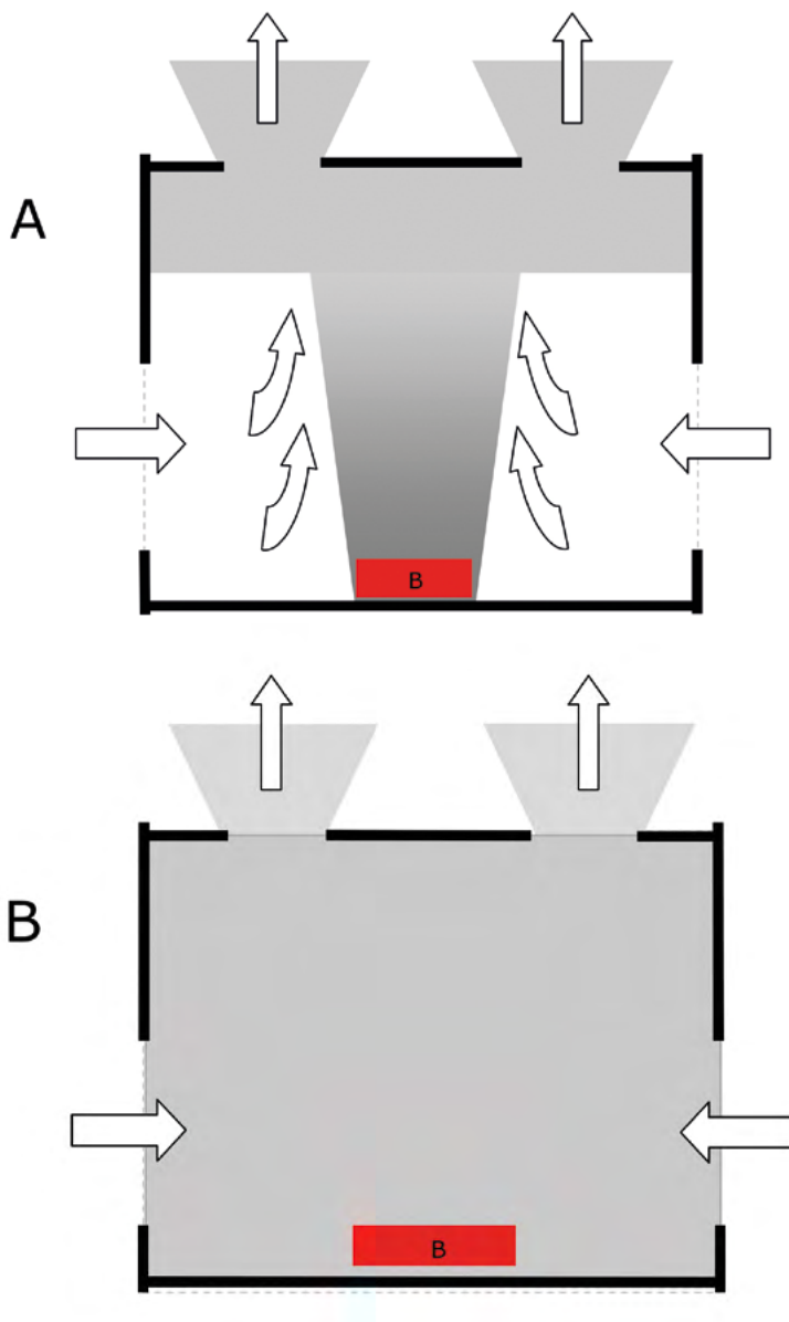
Figuur 38A Schematische weergave van tweezonemodel
