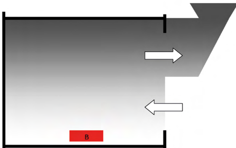
Figuur 37 Schematische weergave van een ventilatiebeheerste brand
